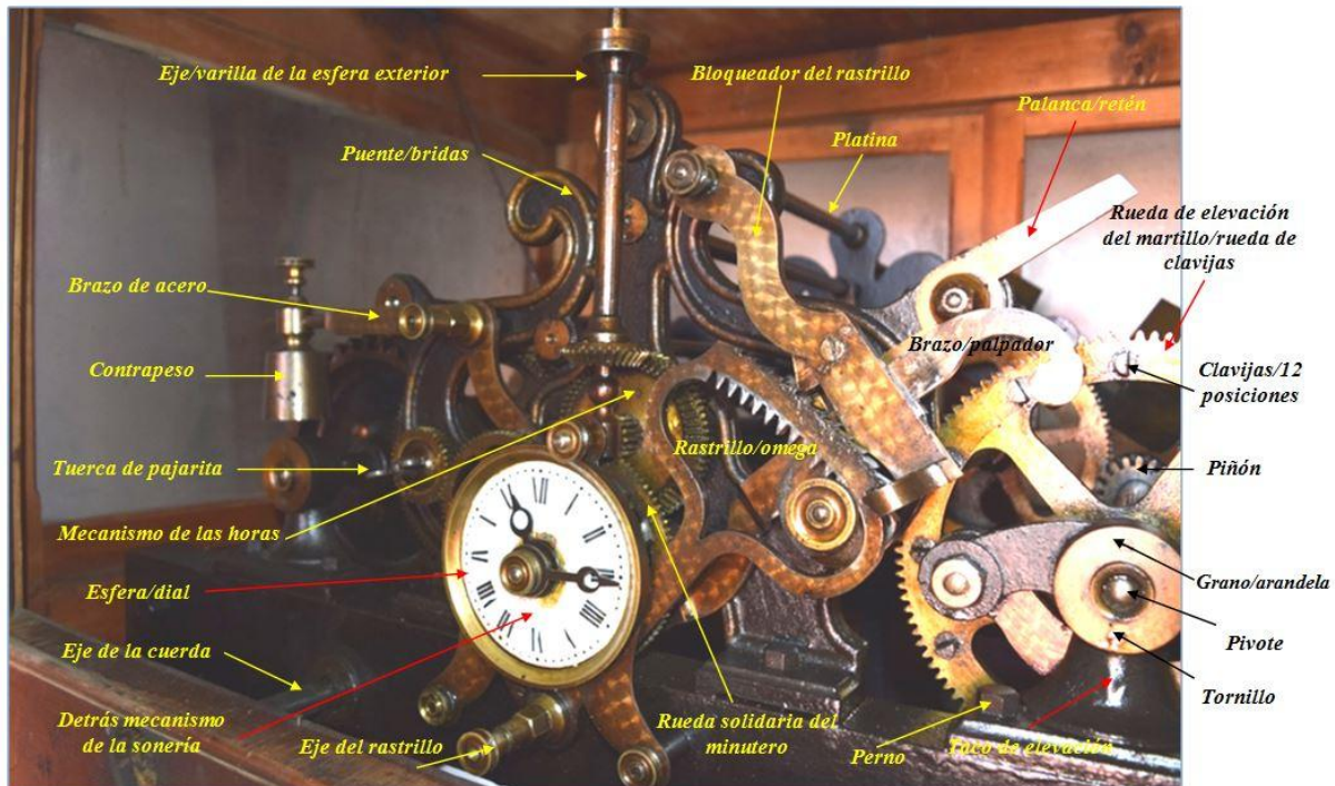
Identificación de algunas partes del mecanismo del reloj público de Agaete. Fotografía realizada por Antonio J. Cruz y Saavedra en marzo de 2019
